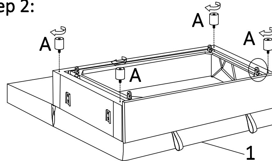
A:LEG 4 PCS
