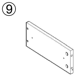
⑨ 300*120*15mm 2PCS
