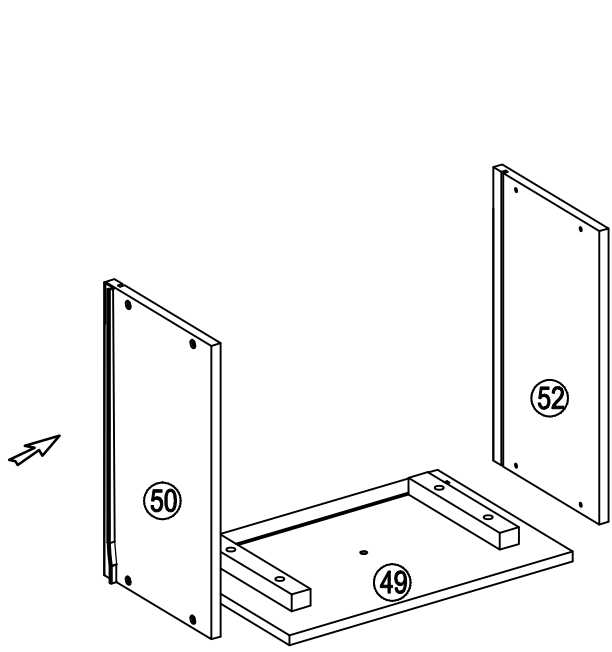
STEP 20
